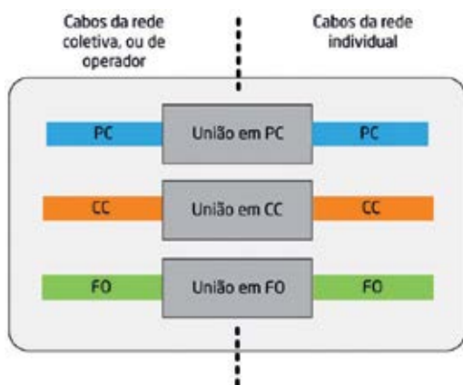
Exemplo de um PTI, fonte Manual ITED 3ª e 4ª Edição.
