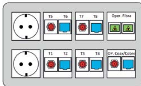
Exemplo de um PCS, fonte Manual ITED 4ª Edição.
